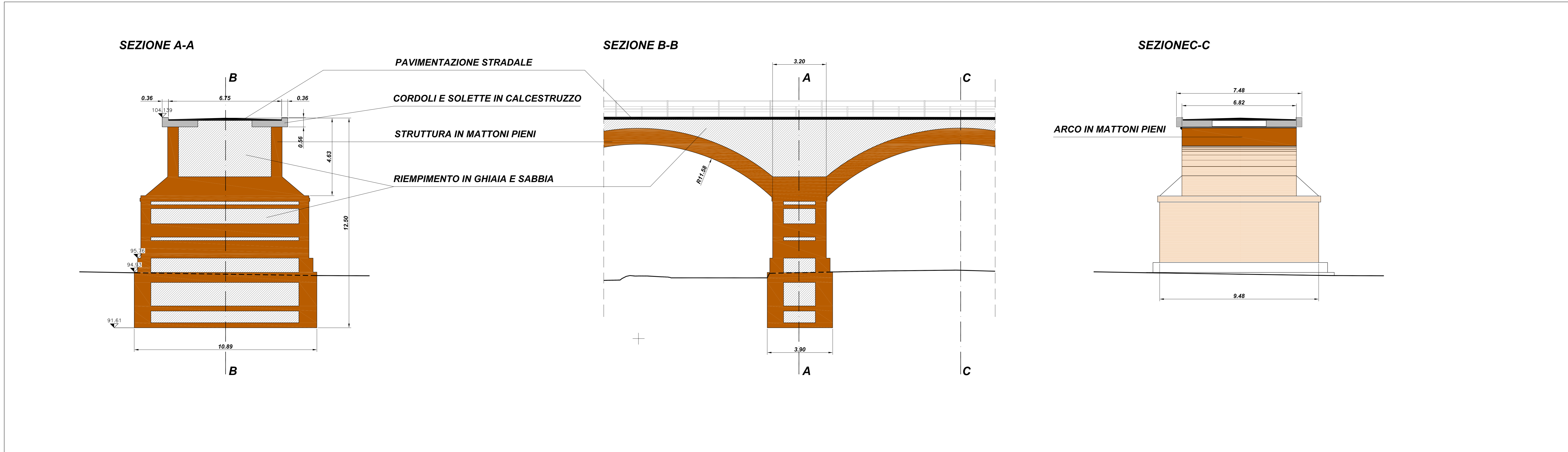
SEZIONI (scala 1:100)
